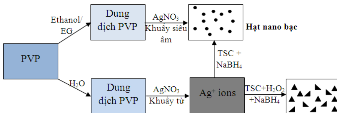
Hình 1. Các quy trình chế tạo hạt nano bạc
